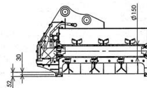
断面図 A-A
