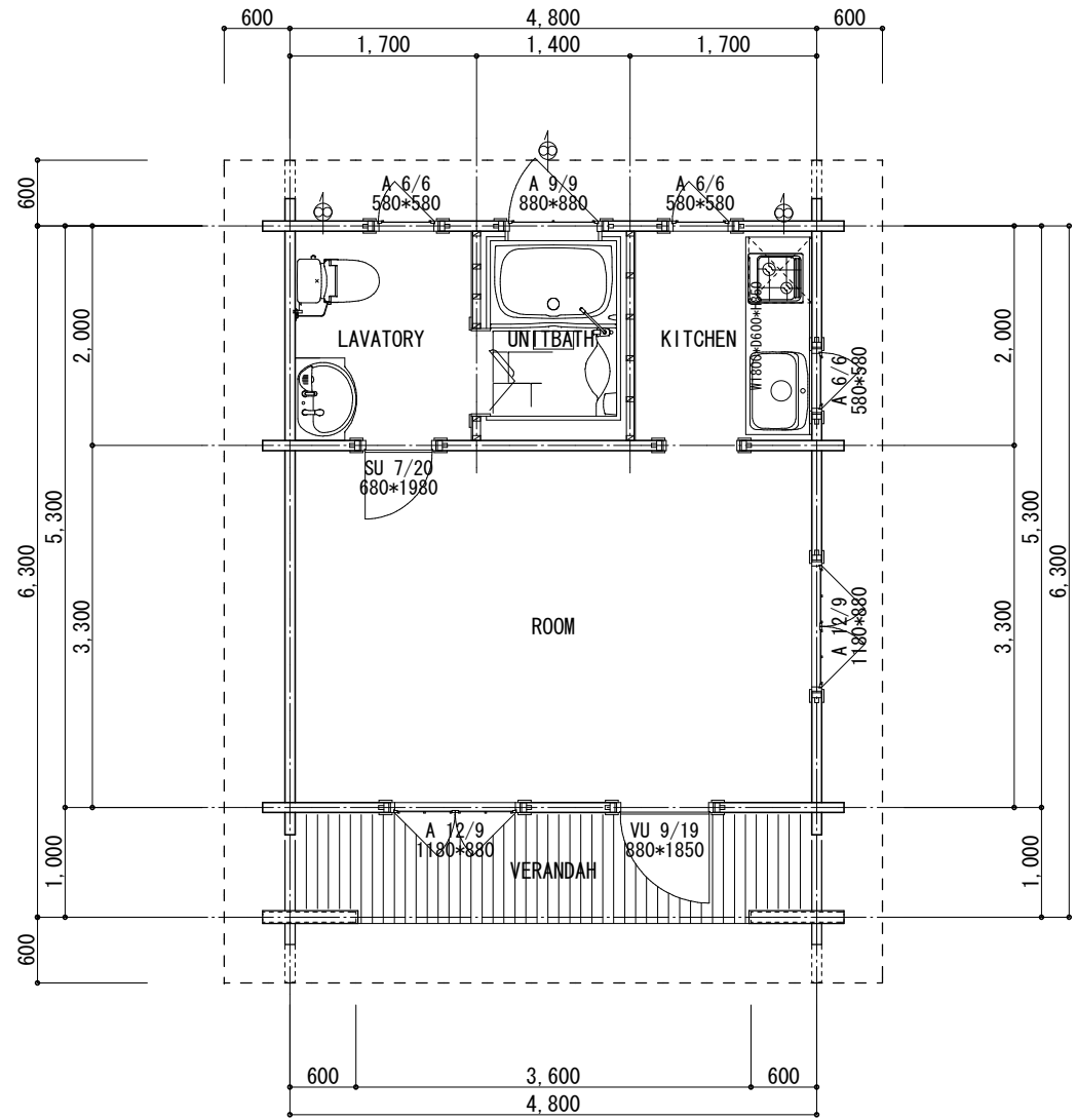
平面図 S=1/50
